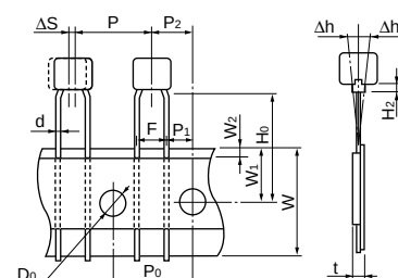
Taping Dimensions
